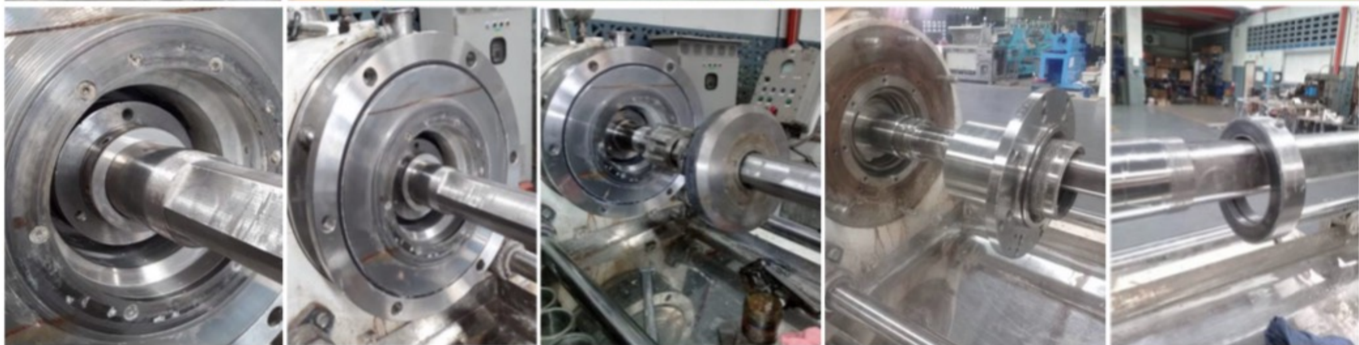
งานซ่อมเครื่องบด Nismix ชุด Mechanical Seal และ Carbide Sieve Ring
